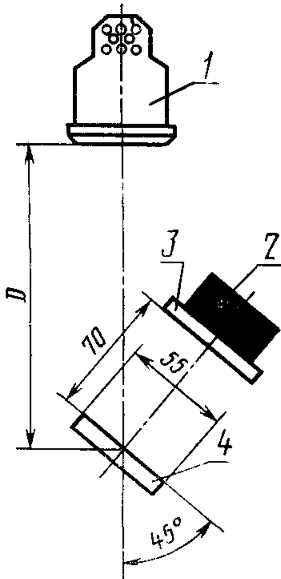
1—ультрафиолетовый облучатель; 2—датчик; 3—светофильтр; 4—люминесцентный экран
